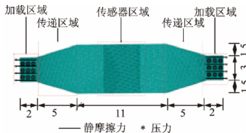
图 8 Abaqus 软件中试件与传感器模型(单位:mm) Fig. 8 Model of specimen and sensor in Abaqus(unit:mm)
