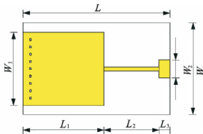
图 4 贴片天线的尺寸
