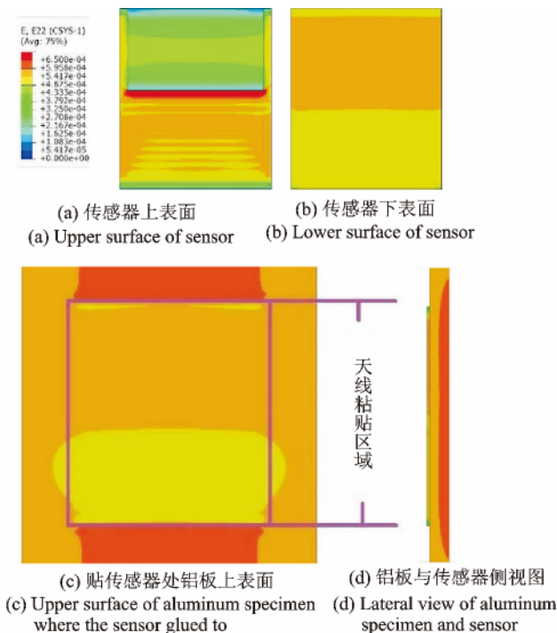
图 9 模型纵向受拉模拟 Fig. 9 Simulation of the longitudinal stretching
