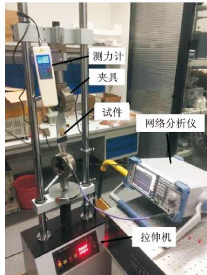
图 12 实验设备
