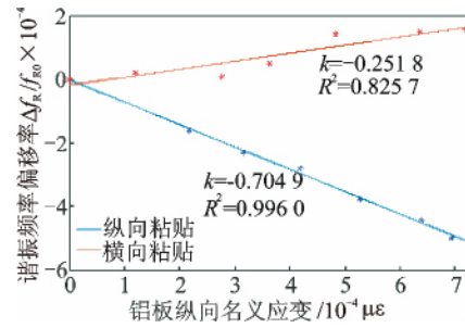
图 14 谐振频率偏移与名义应变的关系实验结果
